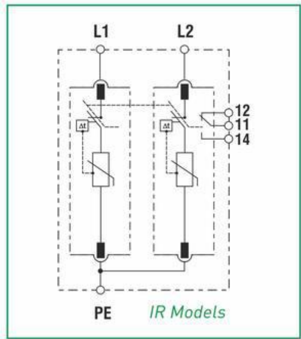
Configuración interna
