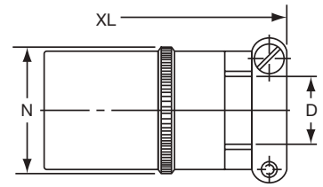
MS3116J-XX-XXX
