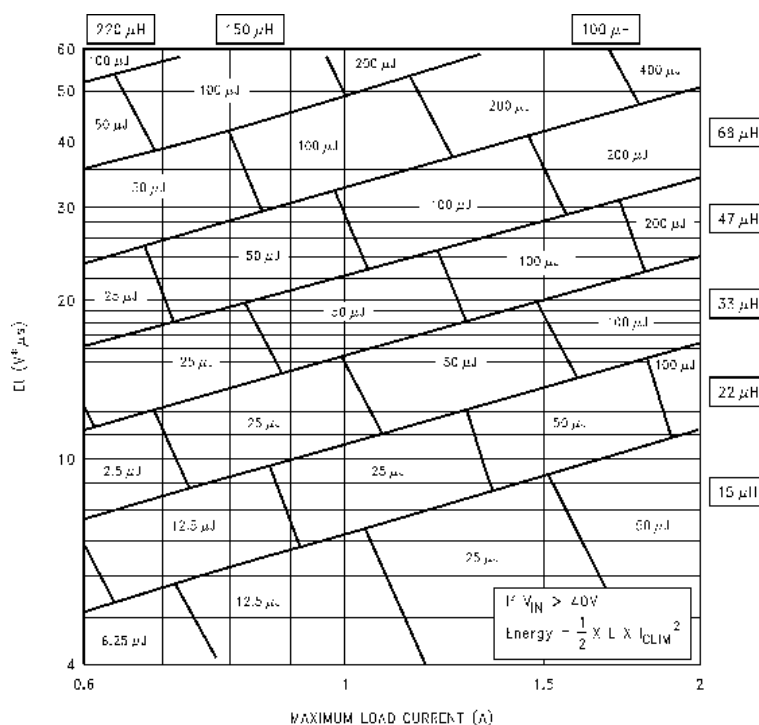
Figure 27. LM2592HV-ADJ
