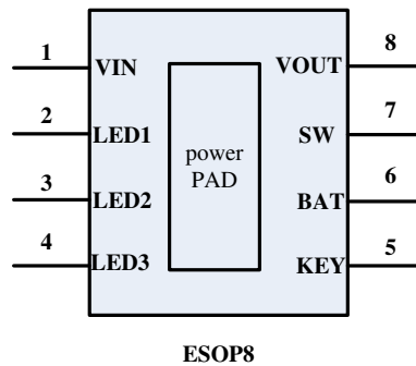
图 2 IP5305/IP5305T 引脚图
