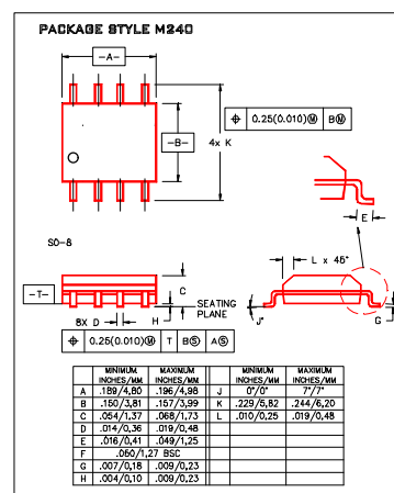
SO-8
